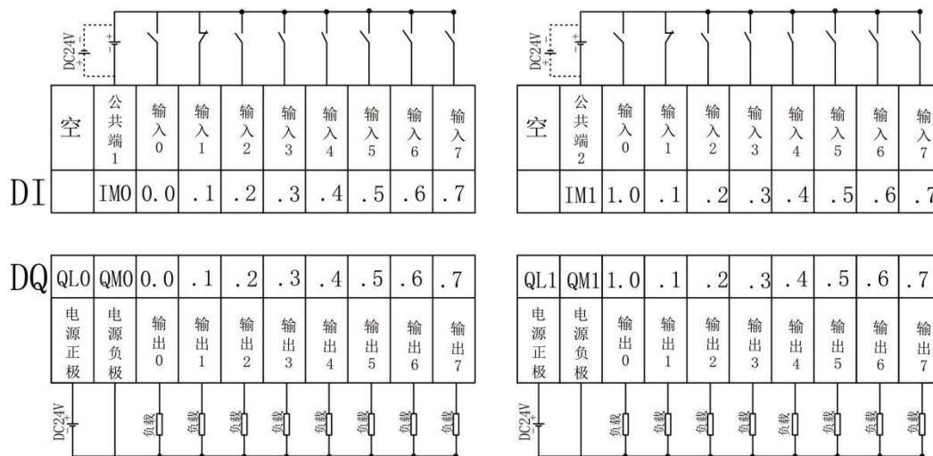
图 3 模块接线图
