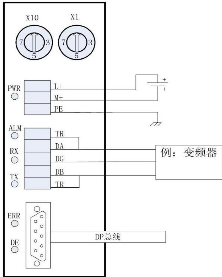
图 2: APG1501 接线图
